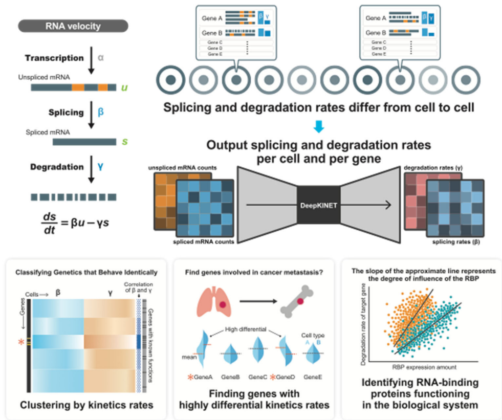
図1 DeepKINETの概要
